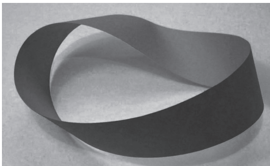
103. ábra: Möbius-szalag.
